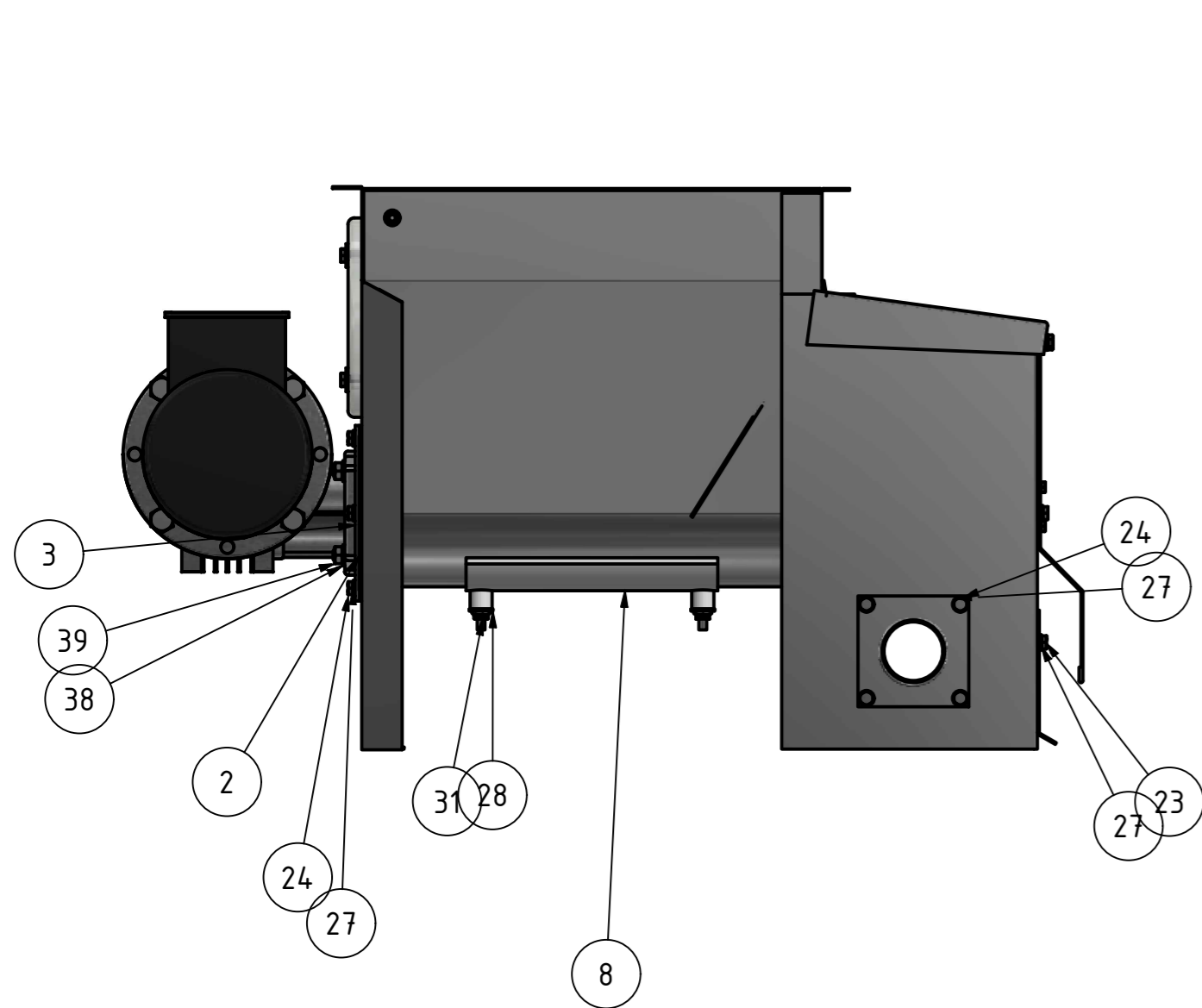
A-A ( 1 : 5 )
