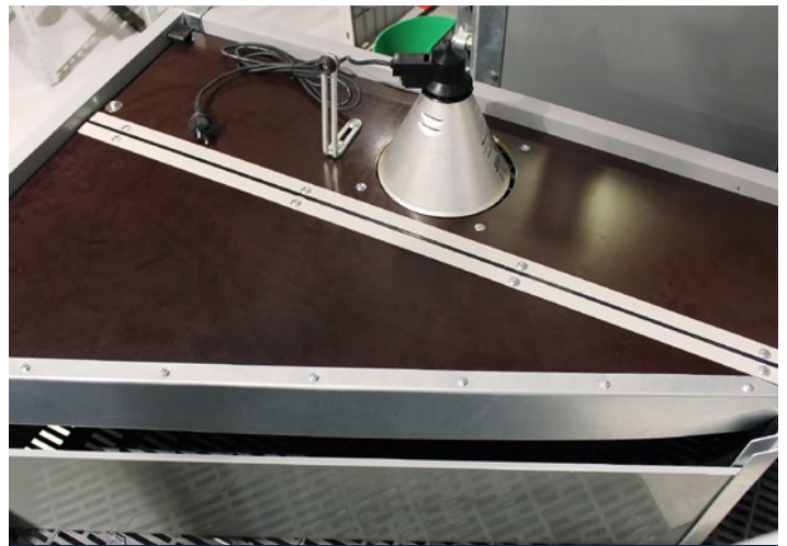
Todelt pattegrisehule med spærreplade og varmelampe
